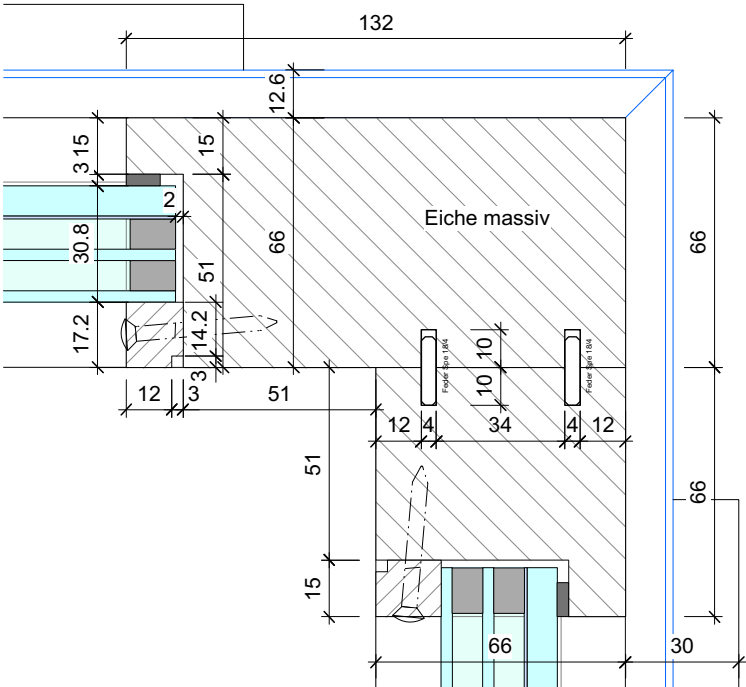
Detail A-A
